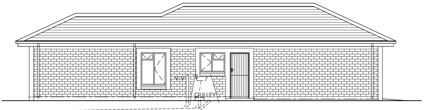
ELEVATION 4
