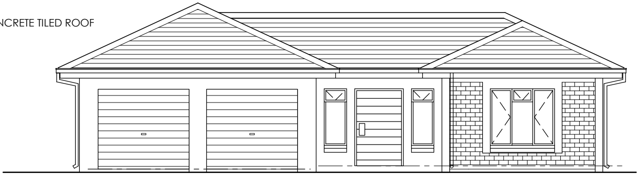
ELEVATION 1
