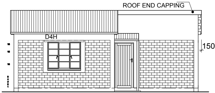
ELEVATION 1
