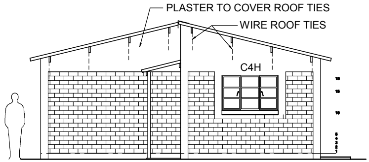
ELEVATION 2
