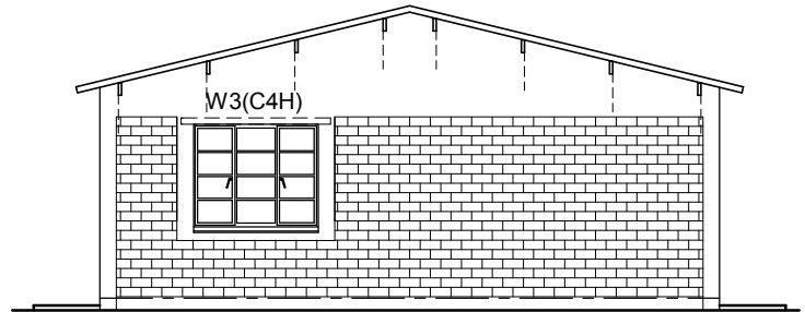
ELEVATION 2
